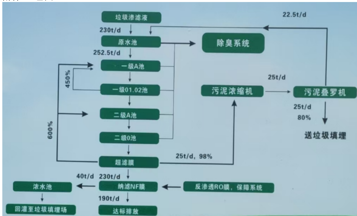
附件1工艺图：
