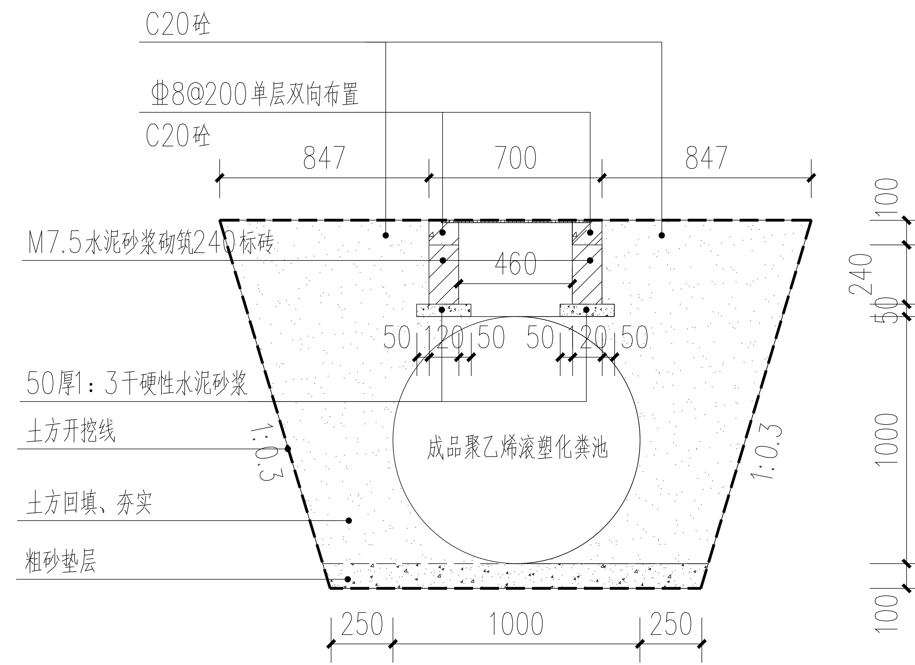
1-1断面图
