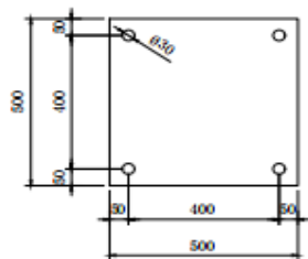
20mm厚预埋板
