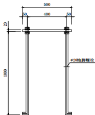
预埋件立面图
