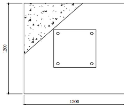
基础平面图
