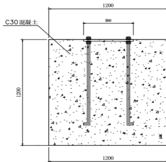
基础立面图
